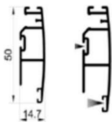
PERFIL MOSQUITERA CORREDERA CURVA
