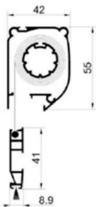
CABEZAL DE 42 mm
